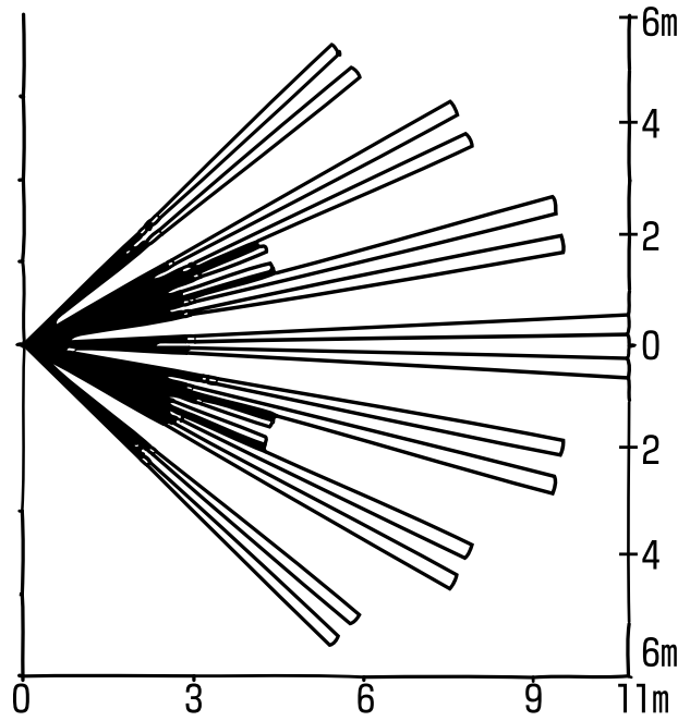
上面図
